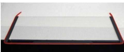
شکل ۵: قرارگیری جداکننده‌های عمودی در دو طرف و جداکننده افقی در پایین ساندویچ ژل Fig. 5: Placing the spacers alongside the inside edges of the gasket
